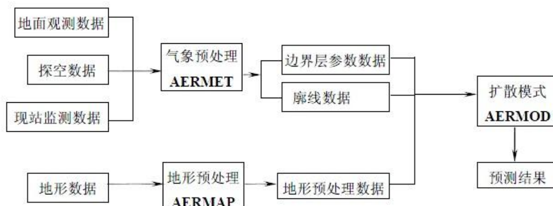
图 6.2-1 AERMOD 模式系统流程图
