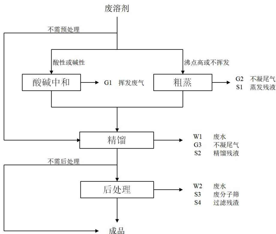
图 4.7-1 废溶剂回收系统工艺流程图
