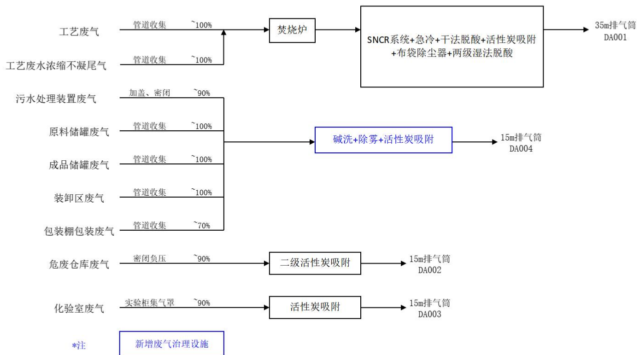
图 7.1-1 本项目废气收集、治理走向图
