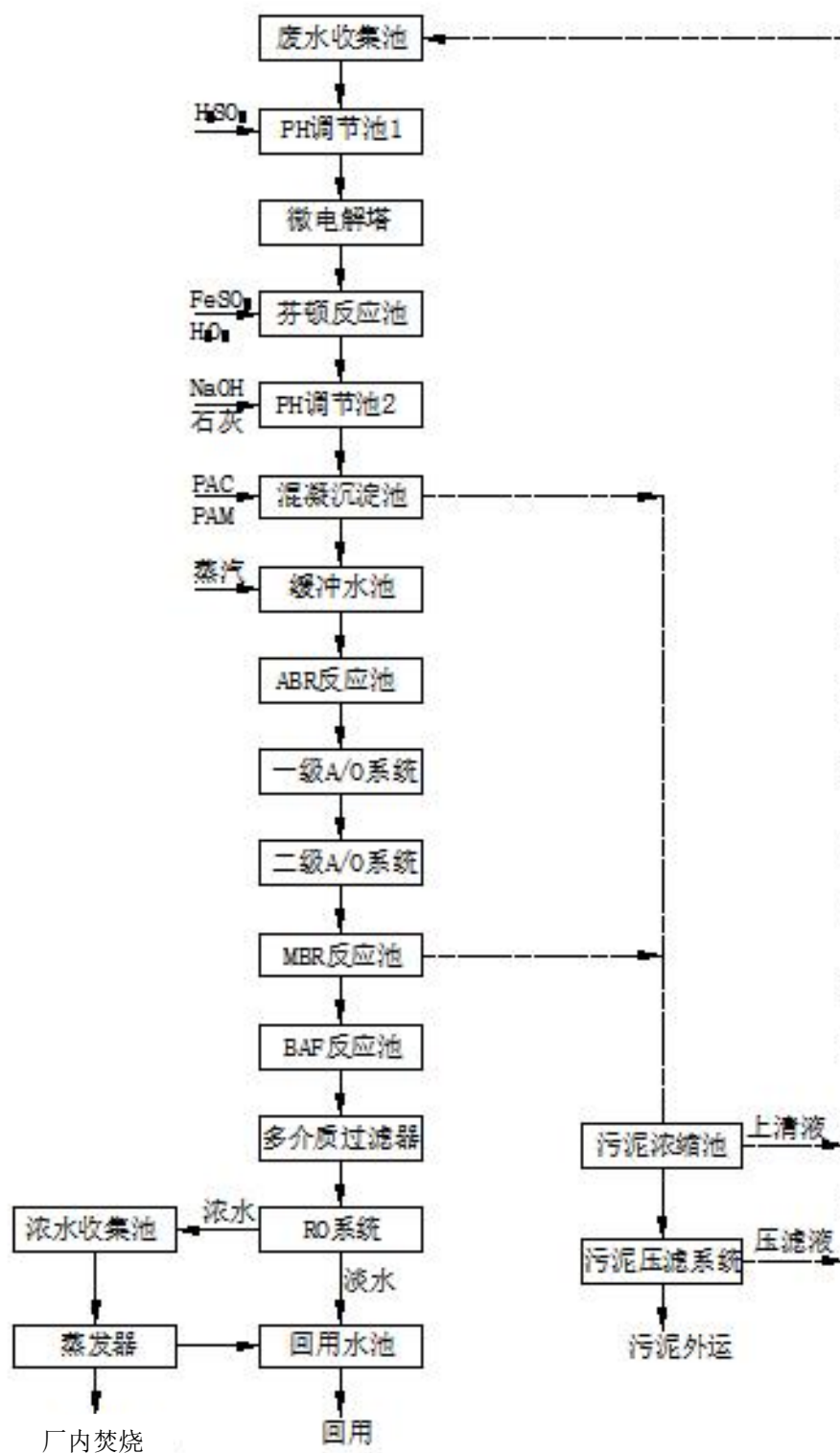
图 7.2-1 本项目废水处理工艺流程图
