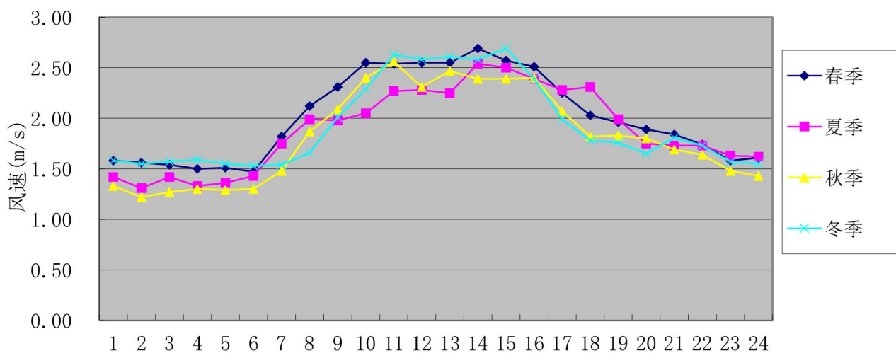
图 6.2-4 季小时平均风速的日变化曲线
