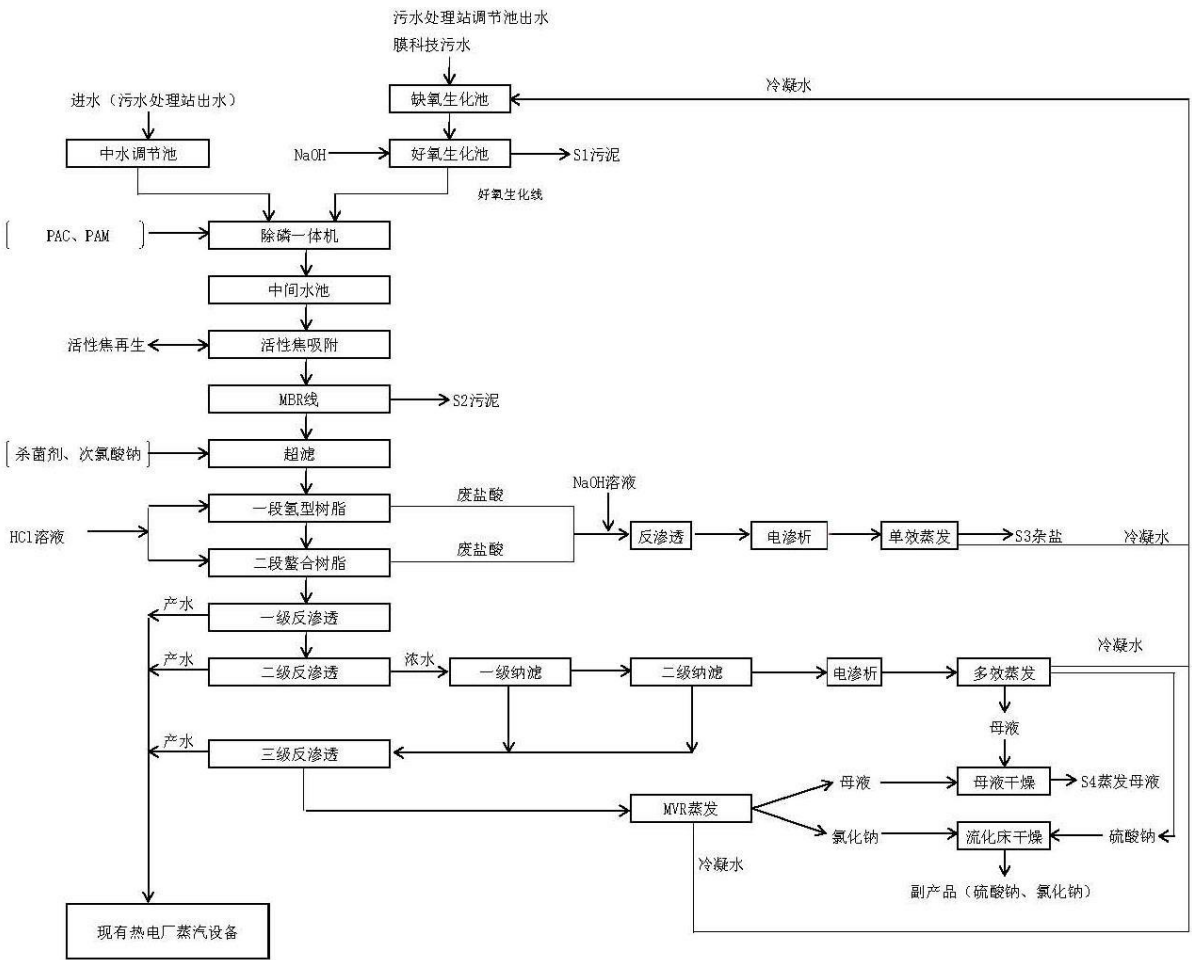
图 7.2-2 富淼废水处理站中水回用零排放处理工艺流程图
