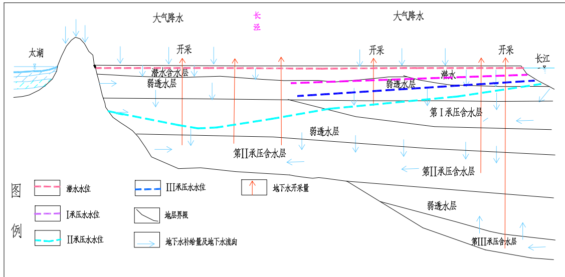
图 6.2-10 研究区各含水层补给和排泄示意图
